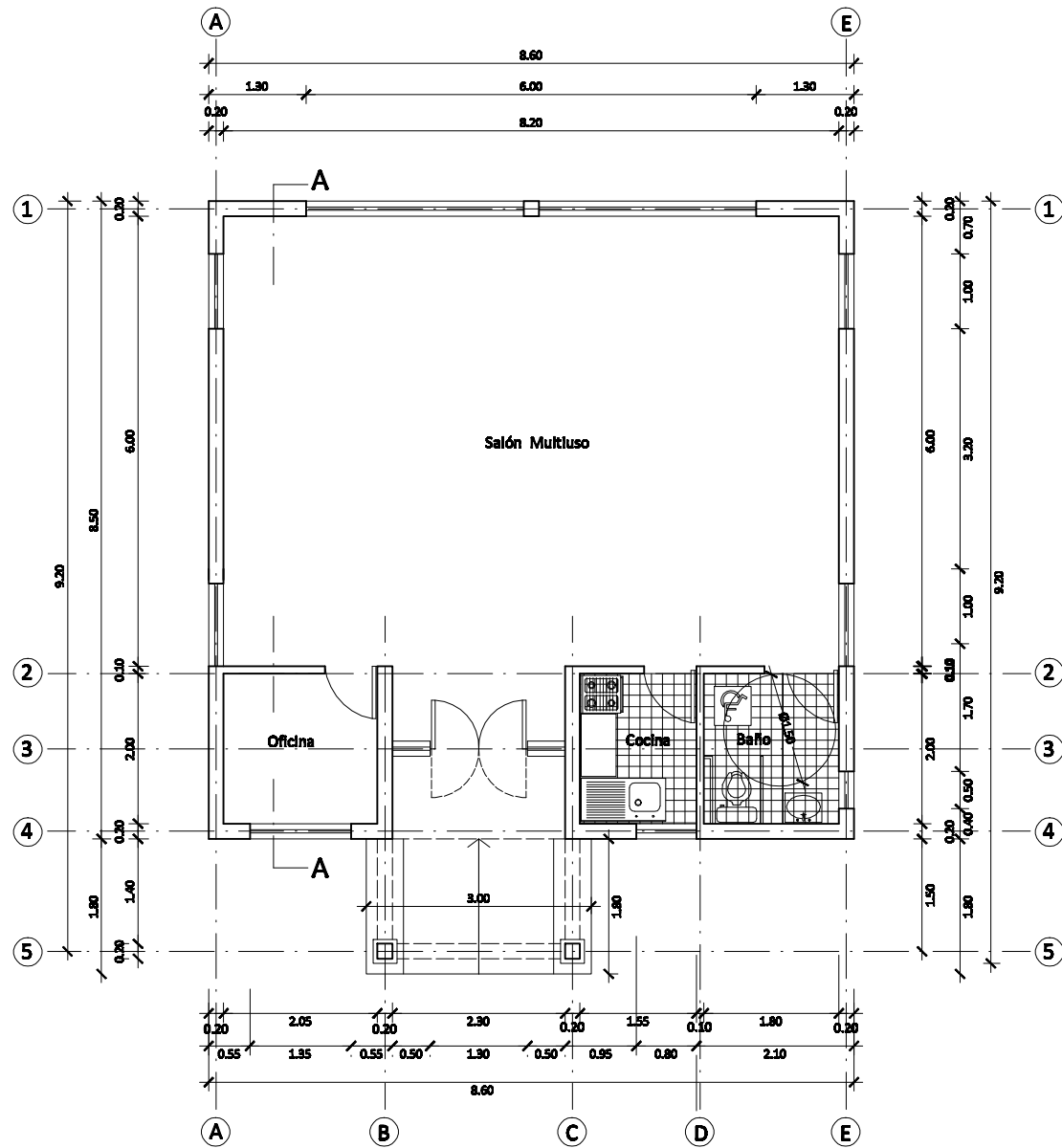
PLANTA DE ARQUITECTURA Esc: 1:50
